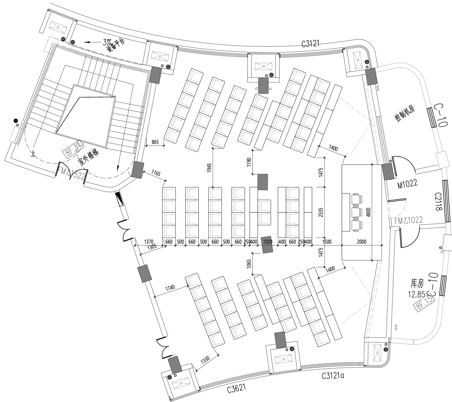
平面布置图
